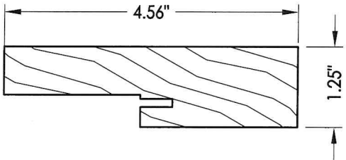
1 HEAD & SIDE JAMB
